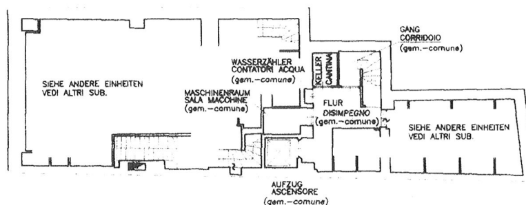
1° KELLERGESCHOSS - 1° PIANO INTERRATO H=2,15-2,20
