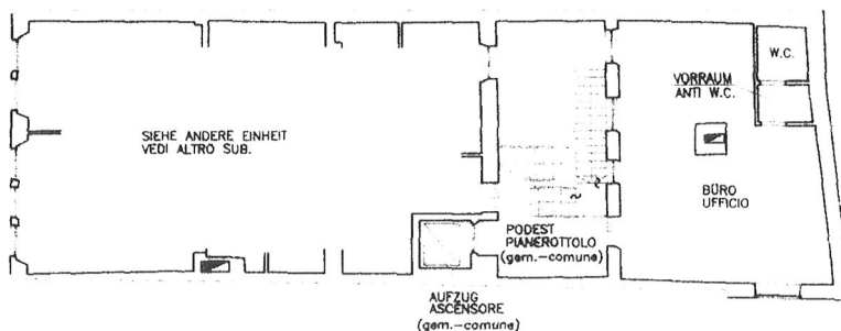
1° OBERGESCHOSS - 1° PIANO H=2,80
